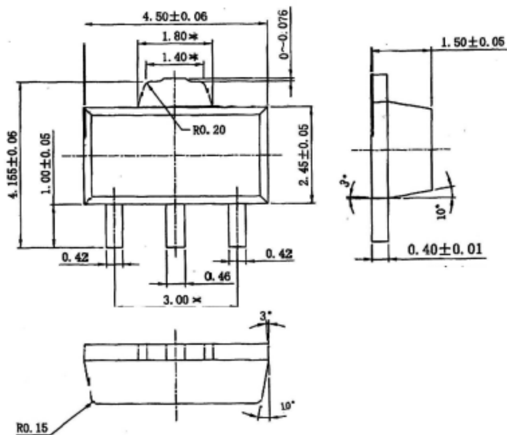
SOT-89-3
